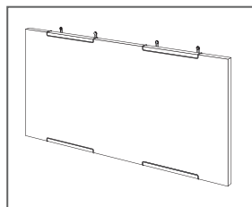
Montaj orizontal pentru Performance Wall C3
