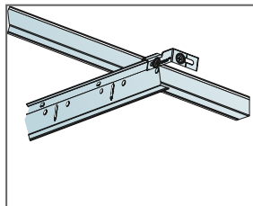
Connect profil principal C4 fixat la perete cu Connect suport de perete C4
