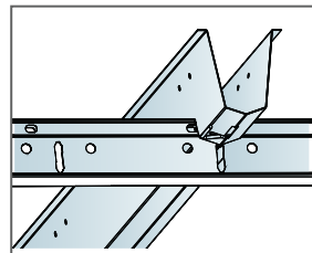
Îmbinarea profilului cu space bar winch
