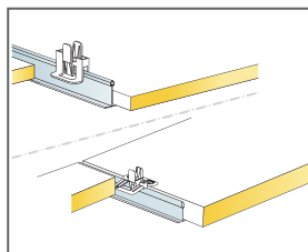
Clemă pentru menținerea plăcilor de 40 mm
