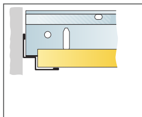
Tăiere dreaptă și profil T deasupra Connect Profil Shadow-line
