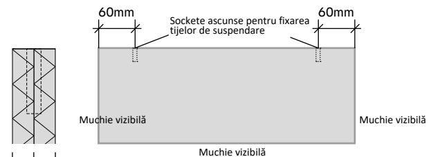
Baffle cu două straturi cu fețe HERADESIGN® și sockete ascunde pentru fixarea tijelor de suspendare livrate.
